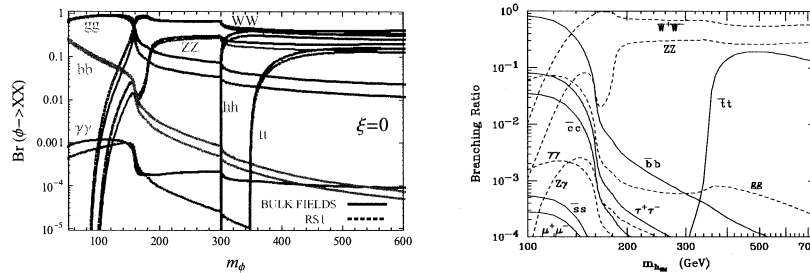
Figure 9: Radion(左図)とヒッグス(右図)の崩壊分岐比の比較。Radion は RS バックグラウンドでのプロットで、実線(点線)はヒッグスがバルク場 (TeV プレーンに局在) に対応。
