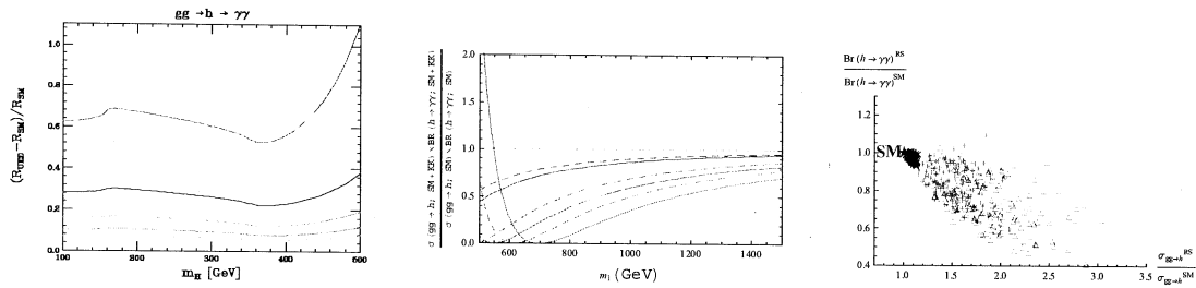
Figure 8: 標準模型と比較した場合の gg \rightarrow H \rightarrow 2\gamma プロセスのイベント数比。UED(左図)、ゲージ・ヒッグス(中央)、RS(右図)。UED では、 R^{-1}=500, 750, 1000, 1250, 1500 GeV の場合のプロット。ゲージ・ヒッグス、RSでは、 m_H = 120 GeV。ゲージ・ヒッグスでは、トップクォークを高い表現に埋め込んだ場合の extra fermion の数が上から n_t = 1, 3, 5 で、実線(点線)は(反)周期境界条件に対応。RSで、 \Delta, +, \times は KK スケールが 1.5, 2, 5 TeV に対応。
