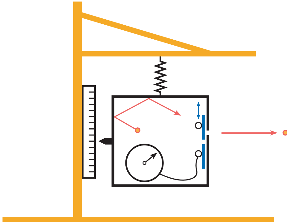
図 1: アインシュタイン・ボーアの光子箱．箱の中には光子が閉じ込められている．箱のシャッターを開けると光子が箱の外に出て行く．シャッターの開閉時刻は時計で測る．また，箱の重さはばね秤で測る．
