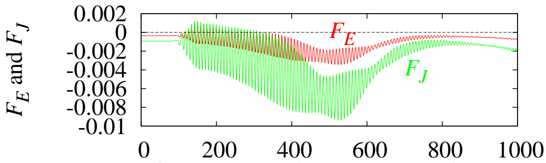
図 6.23: モデル (A): BH ホライズンに落ち込むエネルギーフラックス F_E と角運動量フラックス F_J . 非線形効果はBHからのエネルギーと角運動量の取り出しを増大させる.
