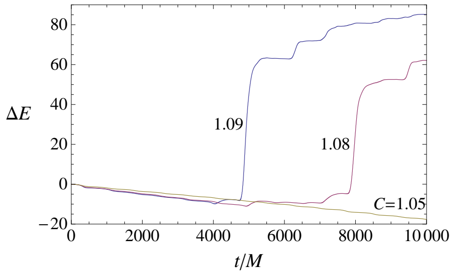
図 6.32: BH に吸収された全エネルギー \Delta E の時間変化. C = 1.05, 1.08, 1.09
