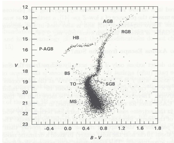
図 4.1: HR 図
