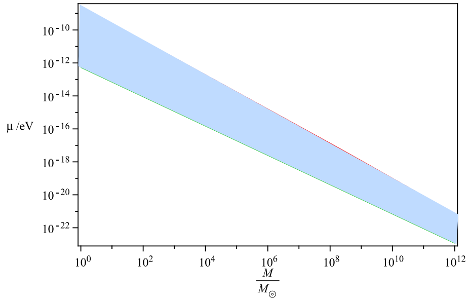
図 6.13: 不安定性成長時間が宇宙年齢以下となる \mu - M の帯状領域
