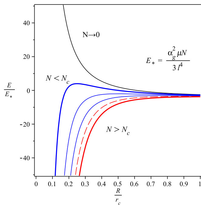
図 6.20: アクシオン雲のエネルギーのサイズ R 依存性
