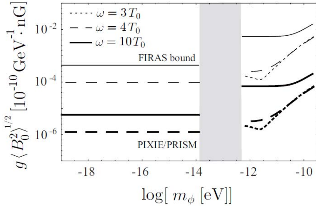
図 5.8: gB への制限
