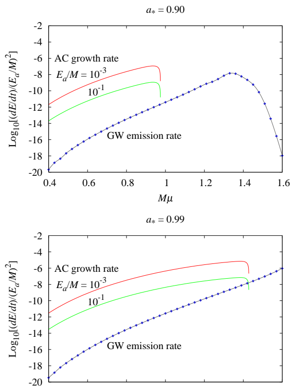
図 6.19: Kerr 時空での GW エネルギー放出率: (\ell, m) = (3, 3) . a_* = 0.90, 0.99 . \tilde{\ell} = 6, 7, 8, 9 .
