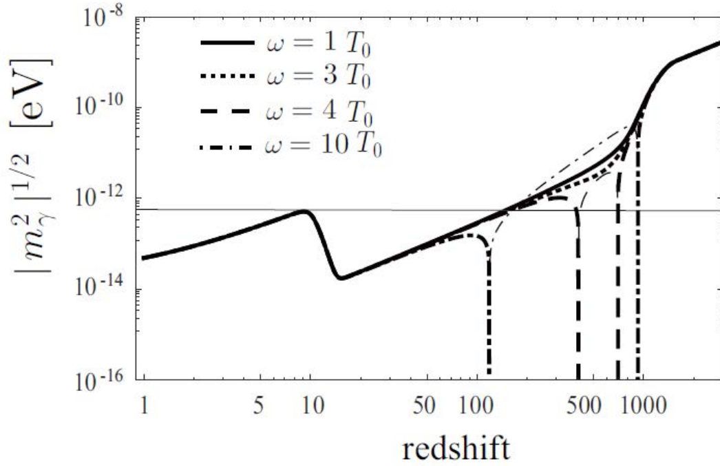
図 5.6: m_\gamma の時間変化
