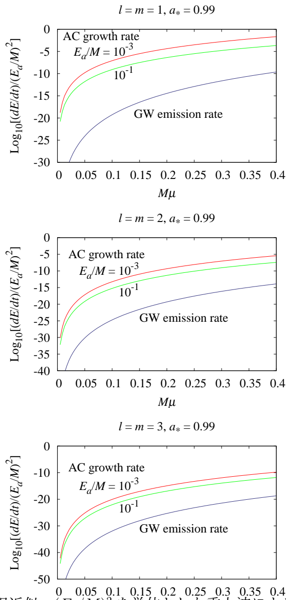
図 6.16: 平坦近似: (E_a/M)^2 を単位とした重力波によるエネルギー放出率とアクシオン増幅反射不安定成長率の比較. \ell = m = 1, 2, 3, n_r = 0, a_* = 0.99 .
