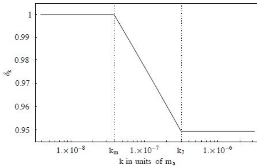
図 5.10: アクシオンによる CDM パワースペクトルの変形
