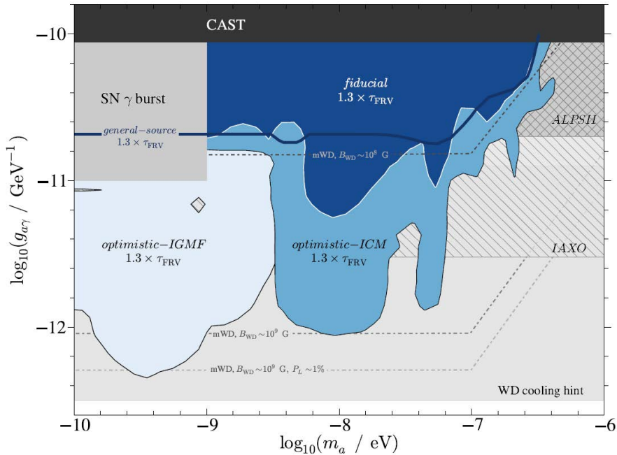
図 4.3: VHE \gamma 線に対する透明度より得られた g_{a\gamma} への下限 [Meyer M, Horns D, Raue M: arXiv:1302.1208]
