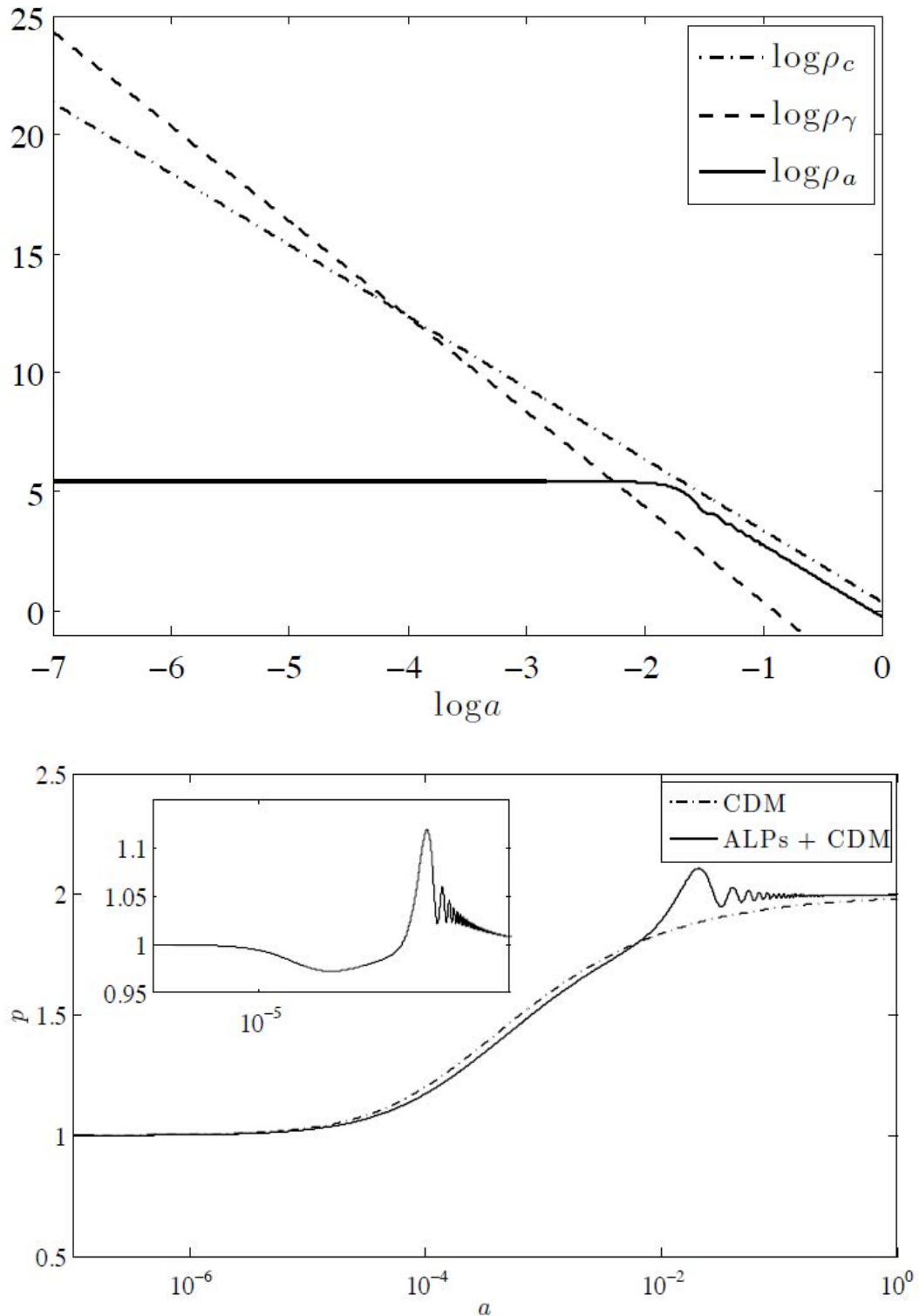
図 5.1: アクシオンのエネルギー密度と膨張指数の時間変化. m/H_0 = 10^3, \Omega_c = 0.8, \Omega_\Lambda = 0 [Marsh DJE, Ferreira PG: PRD82(2010)103528[arXiv:1009.3501]
