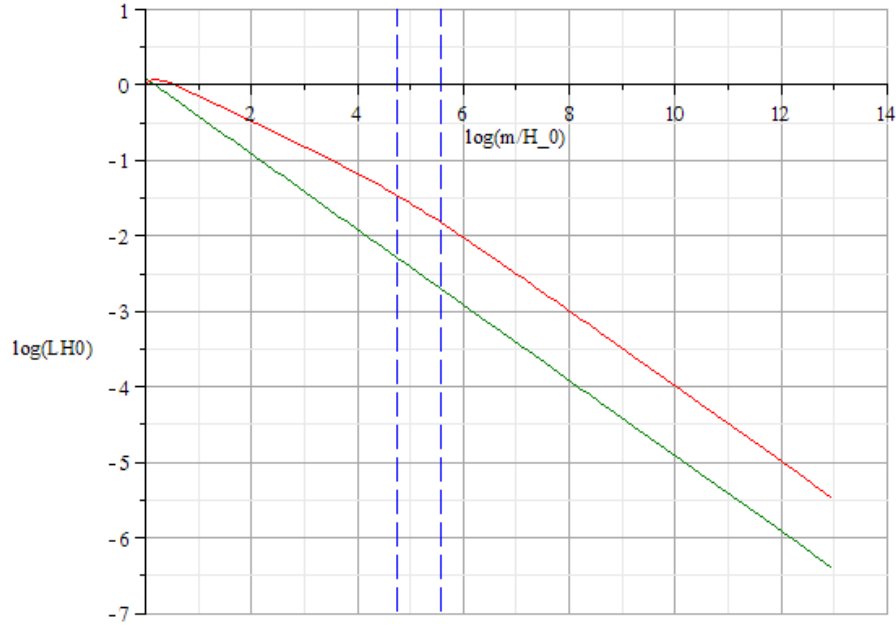
図 5.11: スペクトル変形波長の質量依存性
