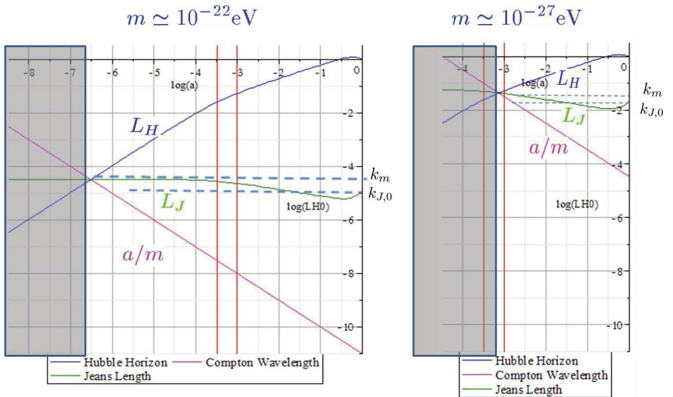
図 5.9: アクシオン Jeans 長の振る舞い
