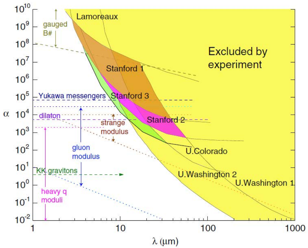
図 3.2: New force への実験的制限 [Geraci AA et al:PRD78(2008)022002]
