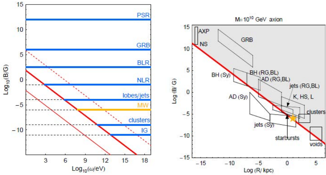
図 4.2: 強いアクシオン・光子混合が起きるための条件
