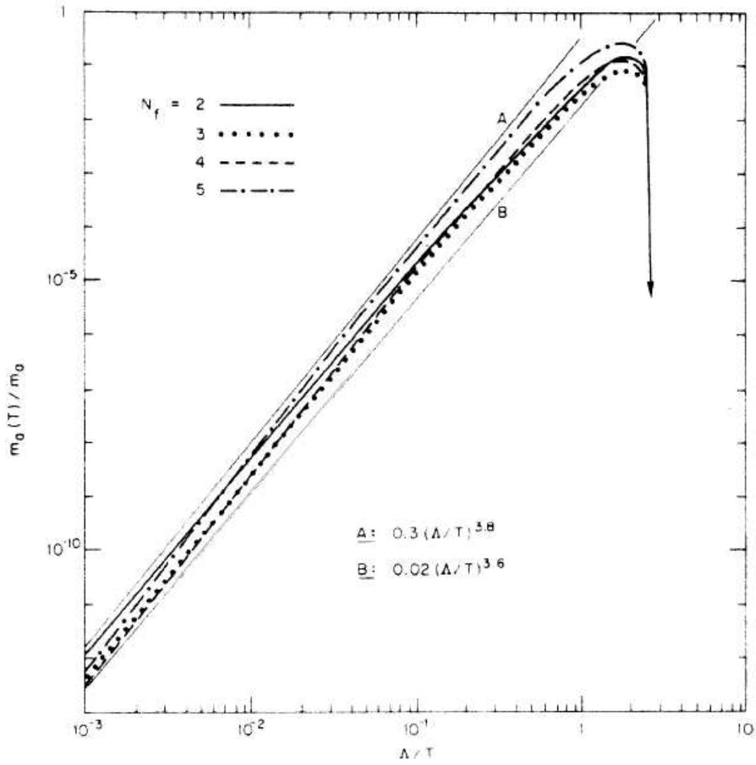
図 5.3: 有限温度でのアクシオン質量
