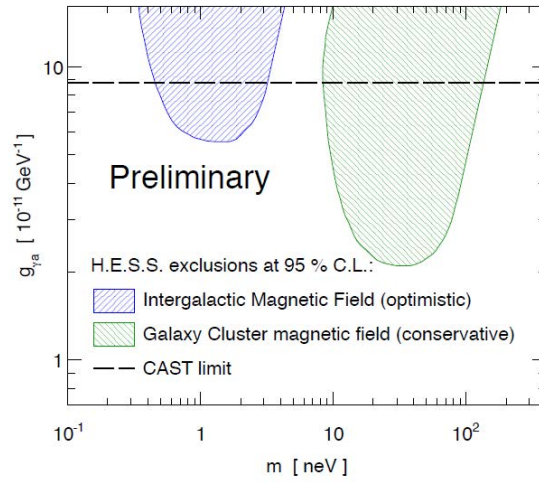
図 4.4: HESS により観測された BL Lac PKS 2155-304 の \gamma 線スペクトルの不規則性より得られた g_{a\gamma} への制限 [Brun P, Wouters D (HESS Collaboration): arXiv: 1307.6068]
