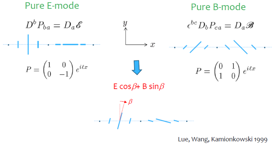
図 5.4: Flat sky 近似での E モードと B モード
