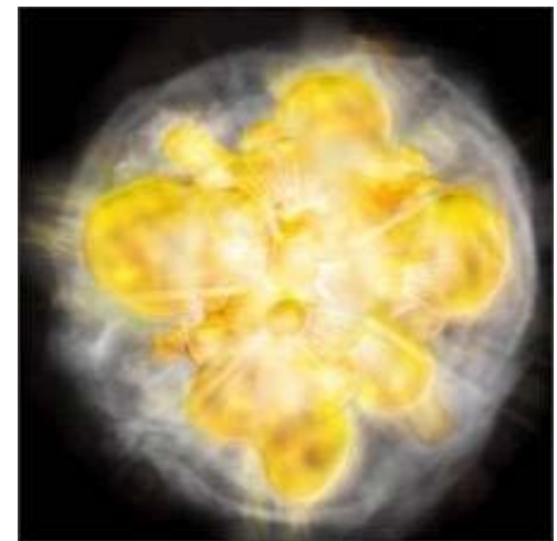
超新星爆発
