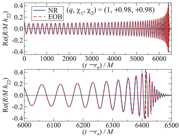
図1 スピンの大きさが共に0.98で、その向きが共に軌道面に垂直方向である場合の等質量の連星ブラックホール合体による重力波の波形。実線が数値相対論の結果を、点線がEOB法による結果を表す。縦に引かれた破線は、振幅最大時の時間を表す。上図が全シミュレーション結果を、下図が合体直前直後の結果を示している。横軸は遅延時間を、縦軸は軌道面に垂直方向から観測した場合の重力波の振幅を表す。Mは2つのブラックホールの質量の和で、時間の単位は GM/c^3 である(Mが太陽質量の20倍ならば、時間の単位は約0.0985ミリ秒)。Rは、重力波源から観測者までの距離を表す。この図では約6,400 GM/c^3 までが公転軌道にある連星からの重力波を表し、それ以後が合体時の重力波を表す。合体後ブラックホールが誕生し定常状態に落ち着く過程で、減衰振動が特徴的な重力波が放射される(下図参照)。文献12から転載。
