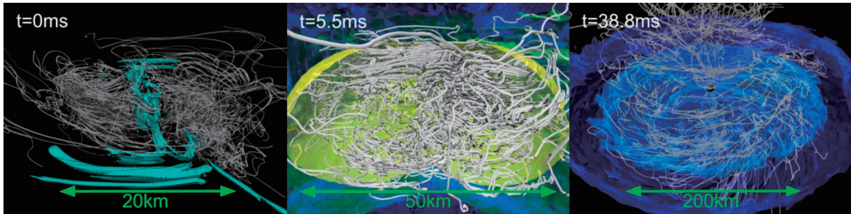
図3 連星中性子星の合体に対する高解像度磁気流体計算の結果。(左) 連星中性子星合体時の磁場強度と磁力線。水色はケルビン・ヘルムホルツ不安定性により急激に磁場が増幅した(磁場強度 10^{15.6} ガウス以上の)領域を、白線は磁力線を表す。(中央) 合体後5.5ミリ秒の密度場の等値面と磁力線(白線)。黄色 = 10^{14} g/cm 3 , 緑 = 10^{12} g/cm 3 , 青 = 10^{10} g/cm 3 を表す。合体後誕生した大質量中性子星の差動回転により、磁場が回転方向に捻られつつ、回転磁気流体不安定性により乱れた磁場が生まれる様子が示されている。(右) 合体後38.8ミリ秒の密度場等値面と磁力線(白線)。青 = 10^{10.5} g/cm 3 , 紺色 = 10^{10} g/cm 3 を表す。中心部にはブラックホールが存在し、その周りに太陽質量の5%程度の質量の、強く磁化された降着円盤が存在する。文献22より転載。
