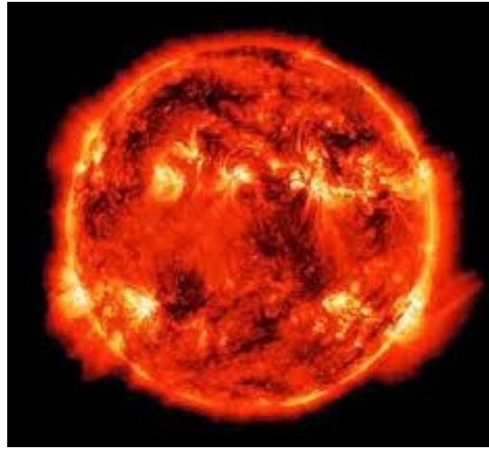
星ができる
