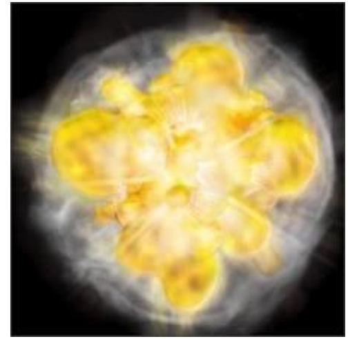
超新星爆発
