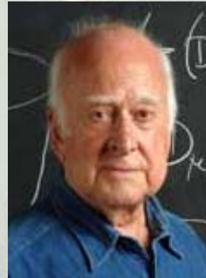
ヒッグス
