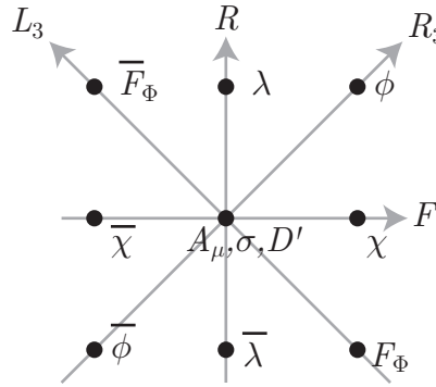
図 2: \mathcal{N} = 4 ベクトル多重項の U(1)_F \times U(1)_R 電荷
