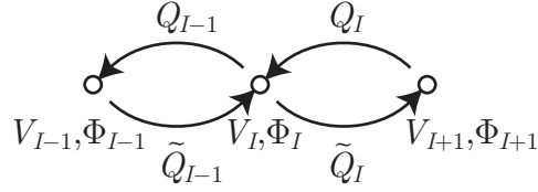
図 12: \mathcal{N} = 4 CS 理論のクイバー図形の一部
