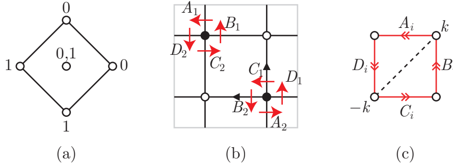
図 24: (a) Q^{1,1,1} のトーリック図形を平面に射影したもの (b) 対応するプレーンタイリング (c) 対応するクイバー CS 理論
